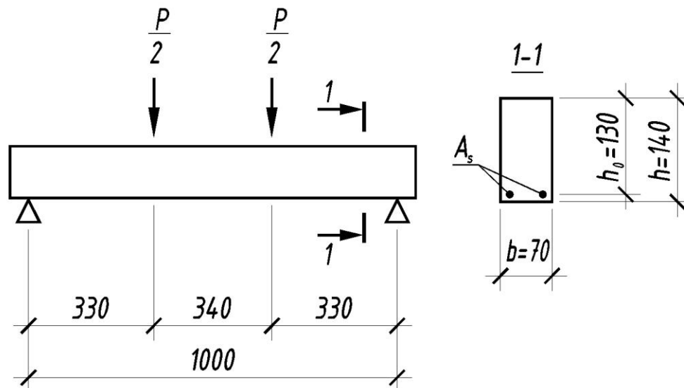
Рисунок 1. Схема испытания и размеры поперечного сечения балки
